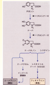
【メラニン生成経路】
